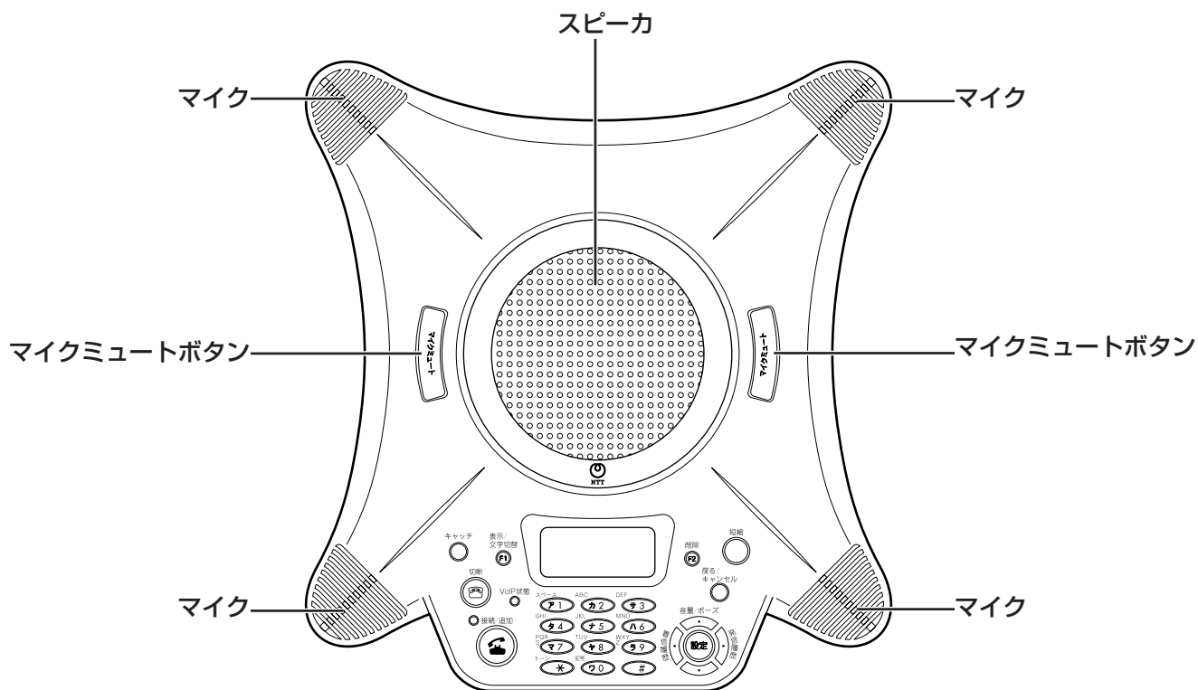
【上面図】
